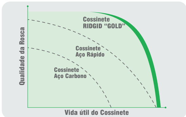
Rosqueado com Cossinetes RIDGID "GOLD"
