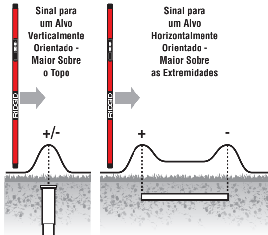
Sinais e Polaridades de Alvos Vertical e Horizontal
